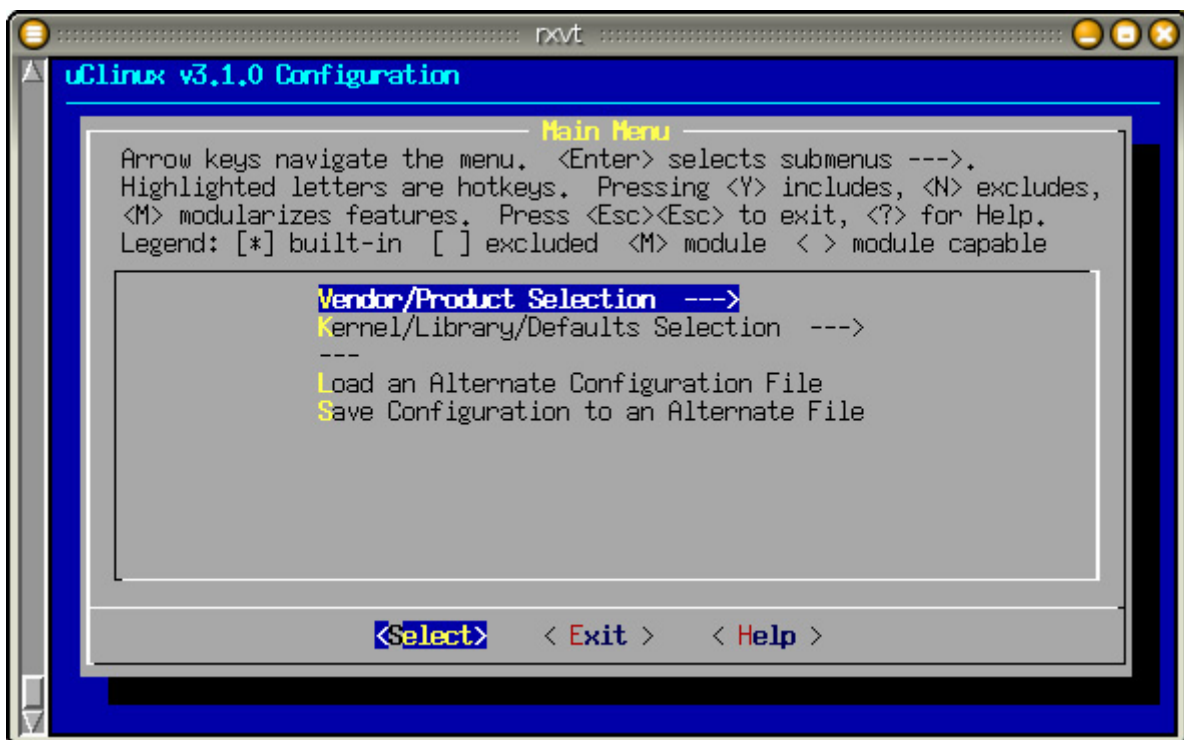
図 6.1. メニューベースコンフィギュレーションの画面
